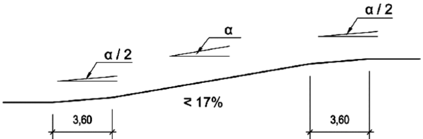
2. ábra: az álláshelyekhez vezető lejtő (közlekedési rámpa)
